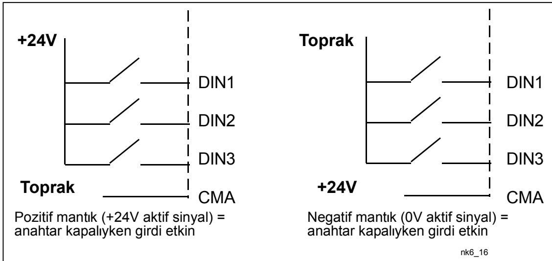
Şekil 6-26. Pozitif/Negatif mantık
