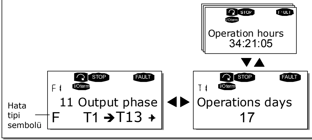
Şekil 7-7. Hata ekranı
