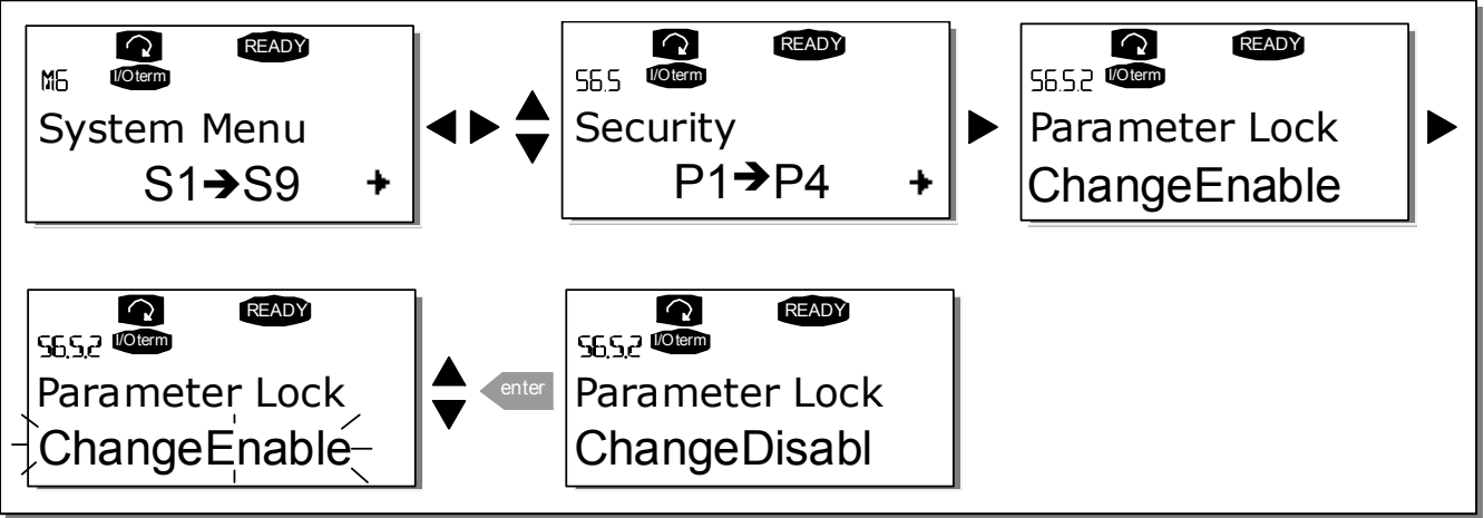
Şekil 7-15. Parametre kilitleme
