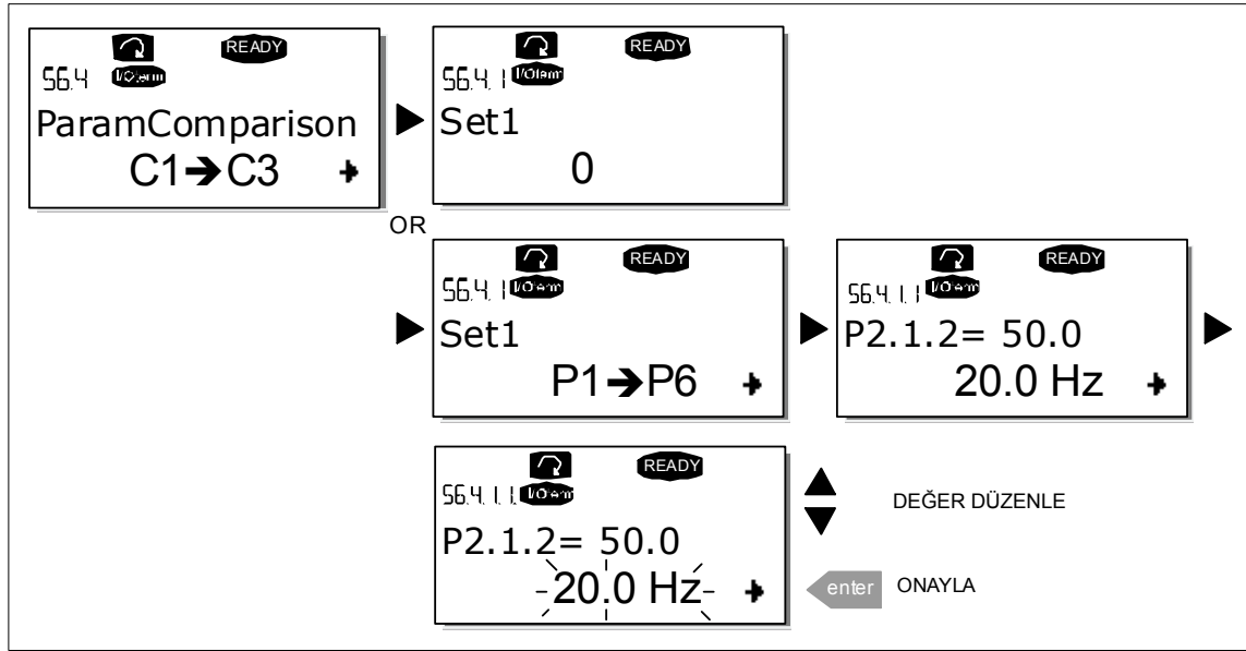
Şekil 7-13. Parametre karşılaştırma
