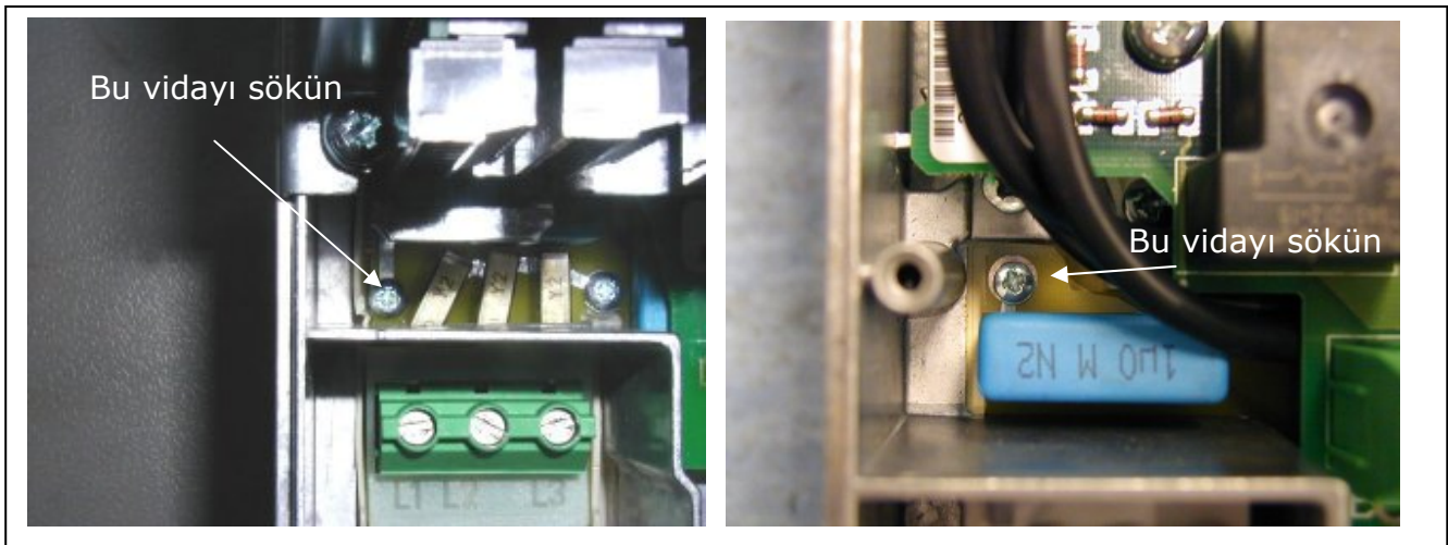
Şekil 5-18. EMC koruma sınıfının değiştirilmesi, FR4 (sol) ve FR5 (sağ).
