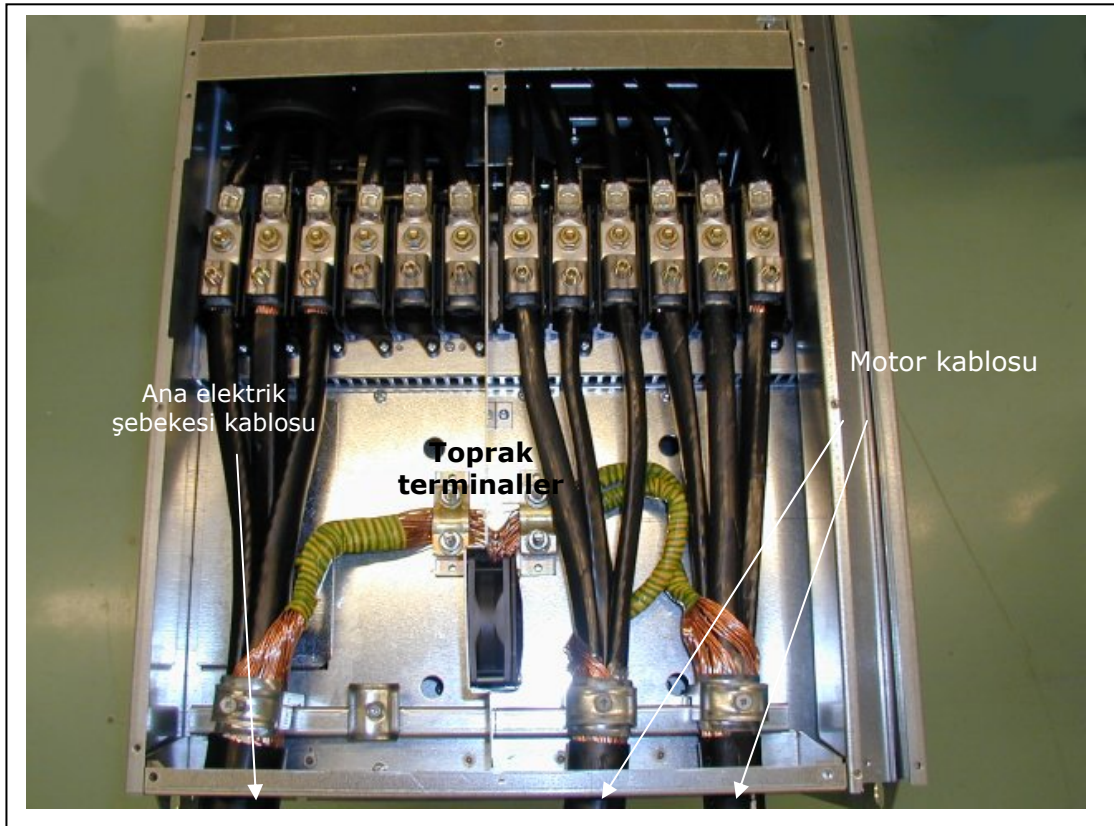
Şekil 6-17. Vacon NX, FR9'de kablo kurulumu
