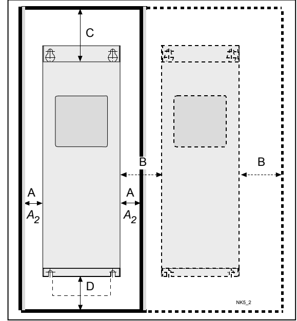
Şekil 5-10. Kurulum alanı
